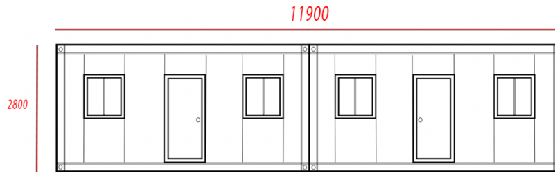
ELEVACIÓN FRONTAL
