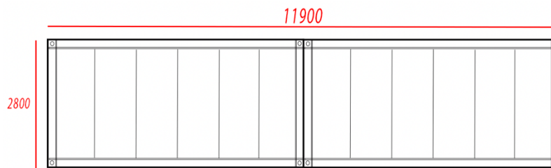
ELEVACIÓN TRASERA
