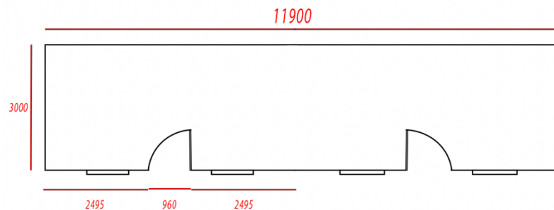
PLANTA BAJA
