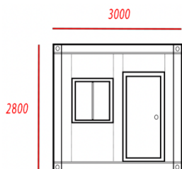
ELEVACION FRONTAL
