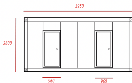
ELEVACION FRONTAL
